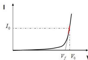
LED特性曲线
